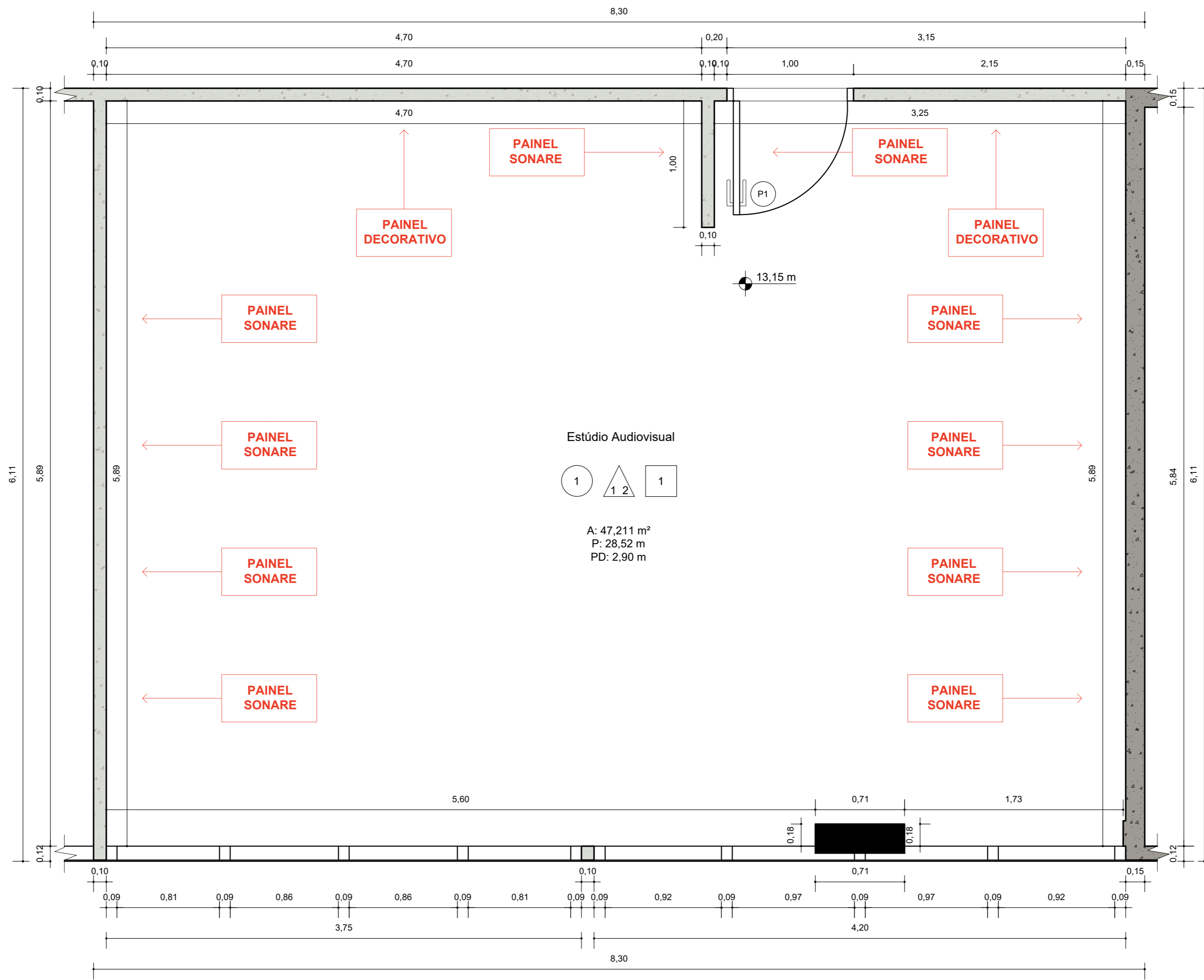
2 PLANTA BAIXA - ESTÚDIO AUDIOVISUAL ESCALA 1:25
